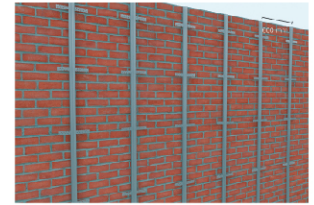
รูปแสดงโครงคร่าวบนผนังก่ออิฐ
