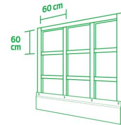
รูปแสดงโครงคร่าวไม้
