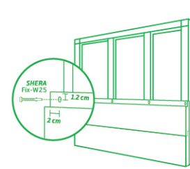
รูปแสดงโครงคร่าวเหล็กชุบสังกะสี
