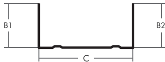
รูปตัดโครงคร่าวตัว "U"
